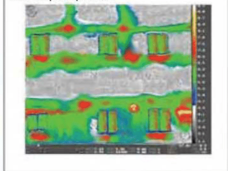
Места промерзания
