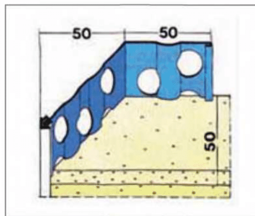
Профиль угловой для армирования углов здания и откосов окон.
