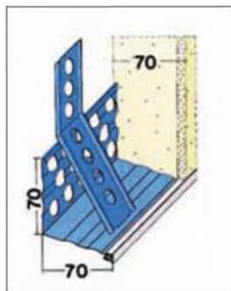
Цокольный профиль
